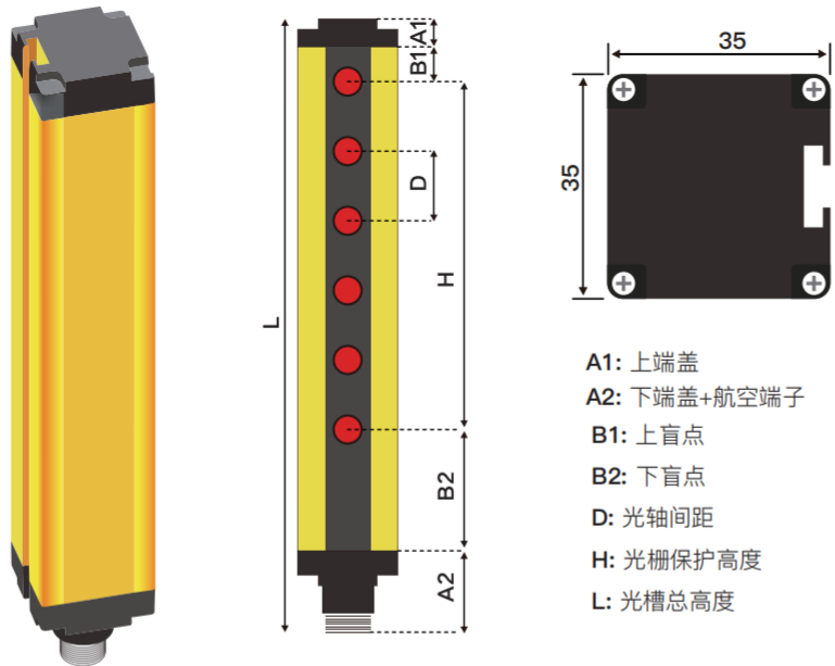
尺寸图
